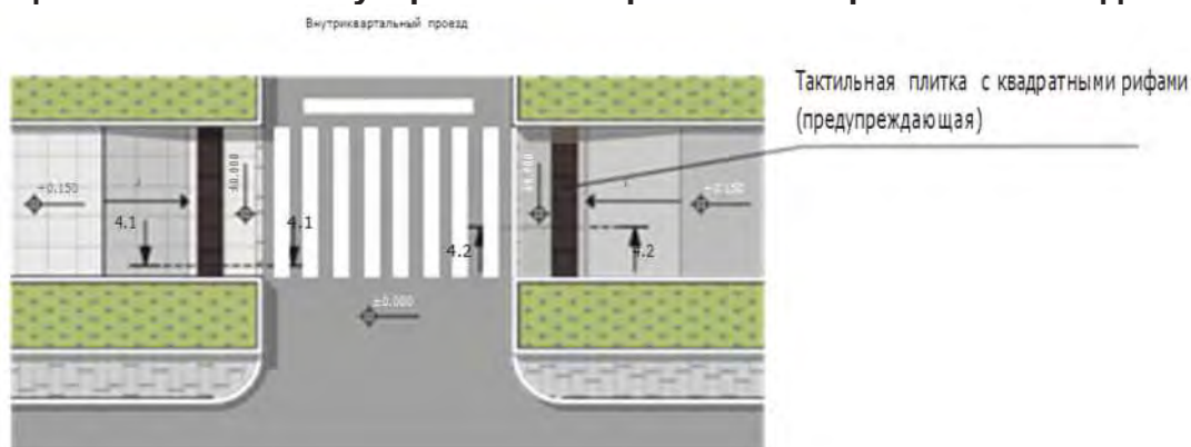
Узел 4.1. Сопряжение тактильной и бетонной плитки (плитки из натурального камня)
