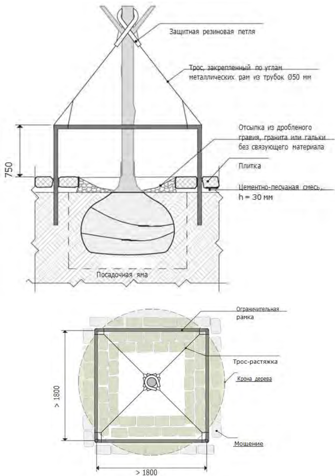
Схема устройства посадочного места в углублении на участке тротуара при закрытой системе орошения и аэрации
