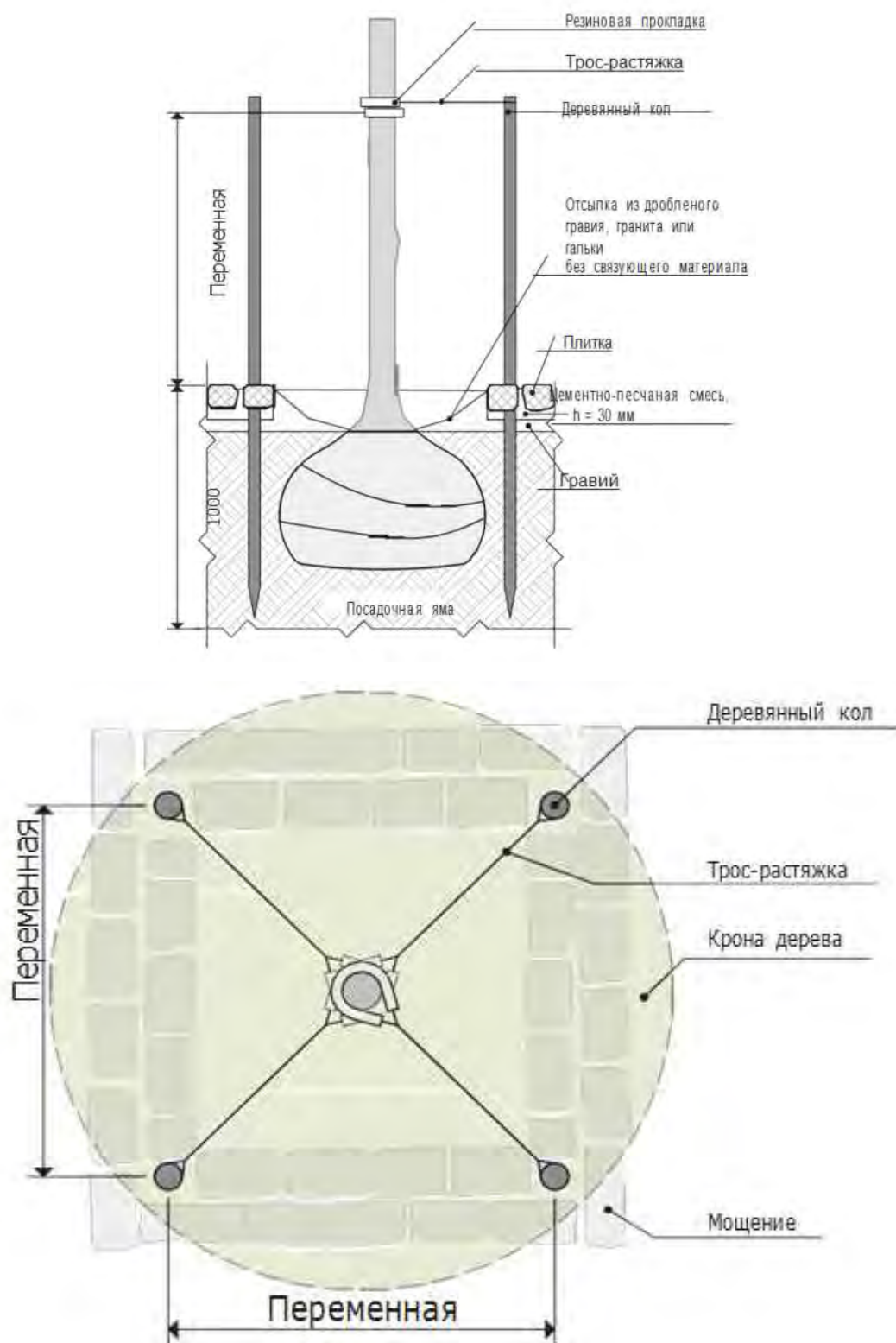
Схема укрепления дерева металлической рамой
