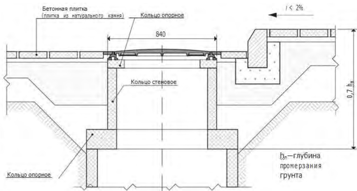
Сечение А–А
