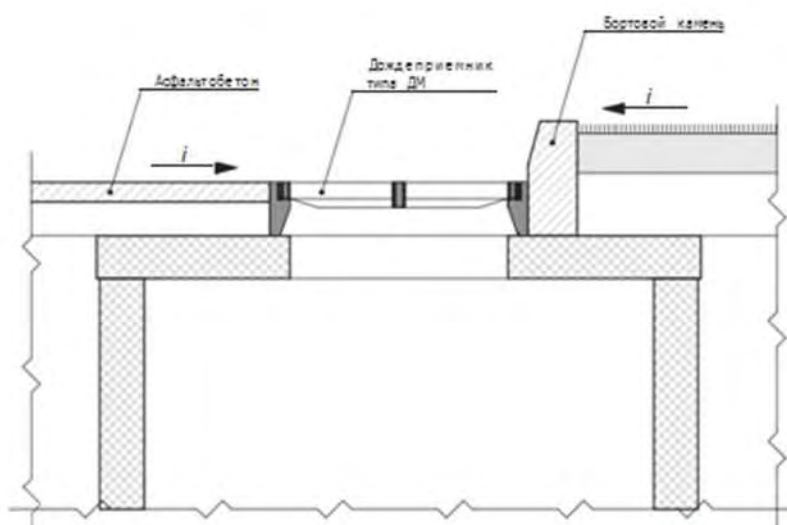
Сечение А-А
