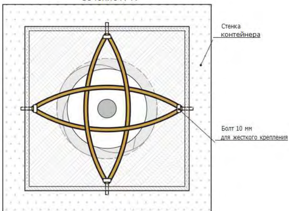
Сечение А-А
